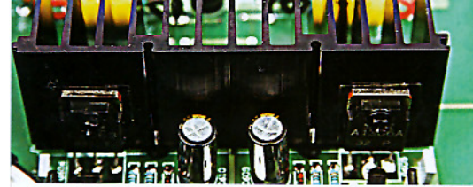
Ένα συμπληρωματικό ζεύγος διπολικών ημιαγωγών βρίσκεται στο στάδιο κέρδους του σταδίου προενίσχυσης.
